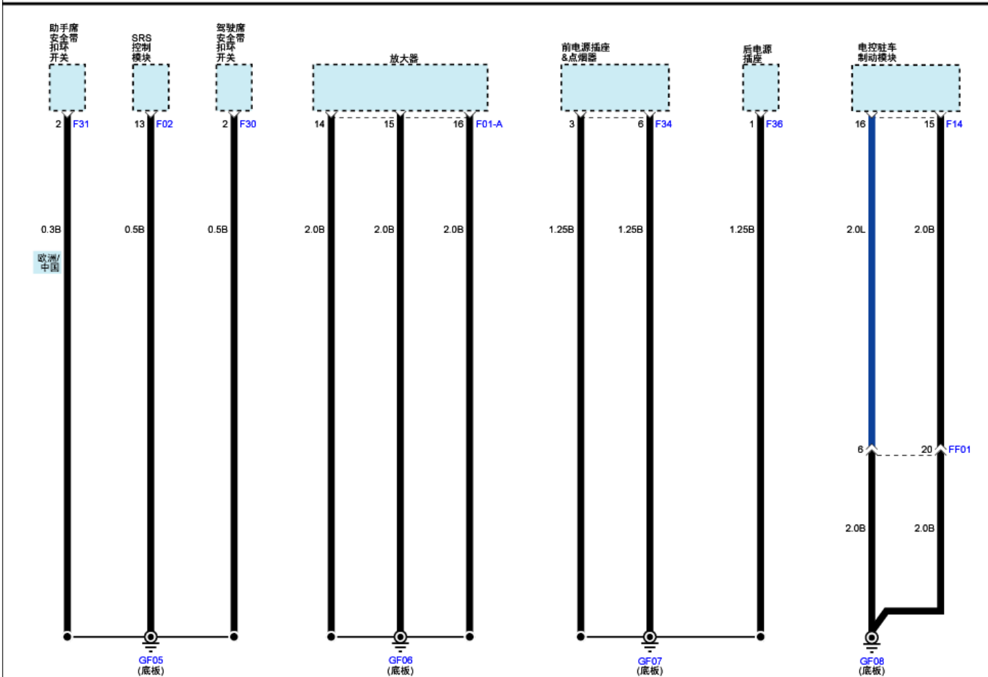
搭铁分布(15)
